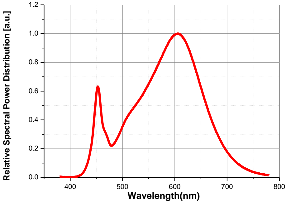
Fig 1. Color Spectrum, T_a=25^\circ\text{C} , I_F=20\text{mA}
